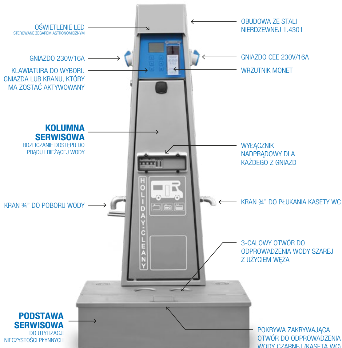
PODSTAWA SERWISOWA USUWANIE NIECZYSTOŚCI PŁYNNYCH Z KASETY WC
